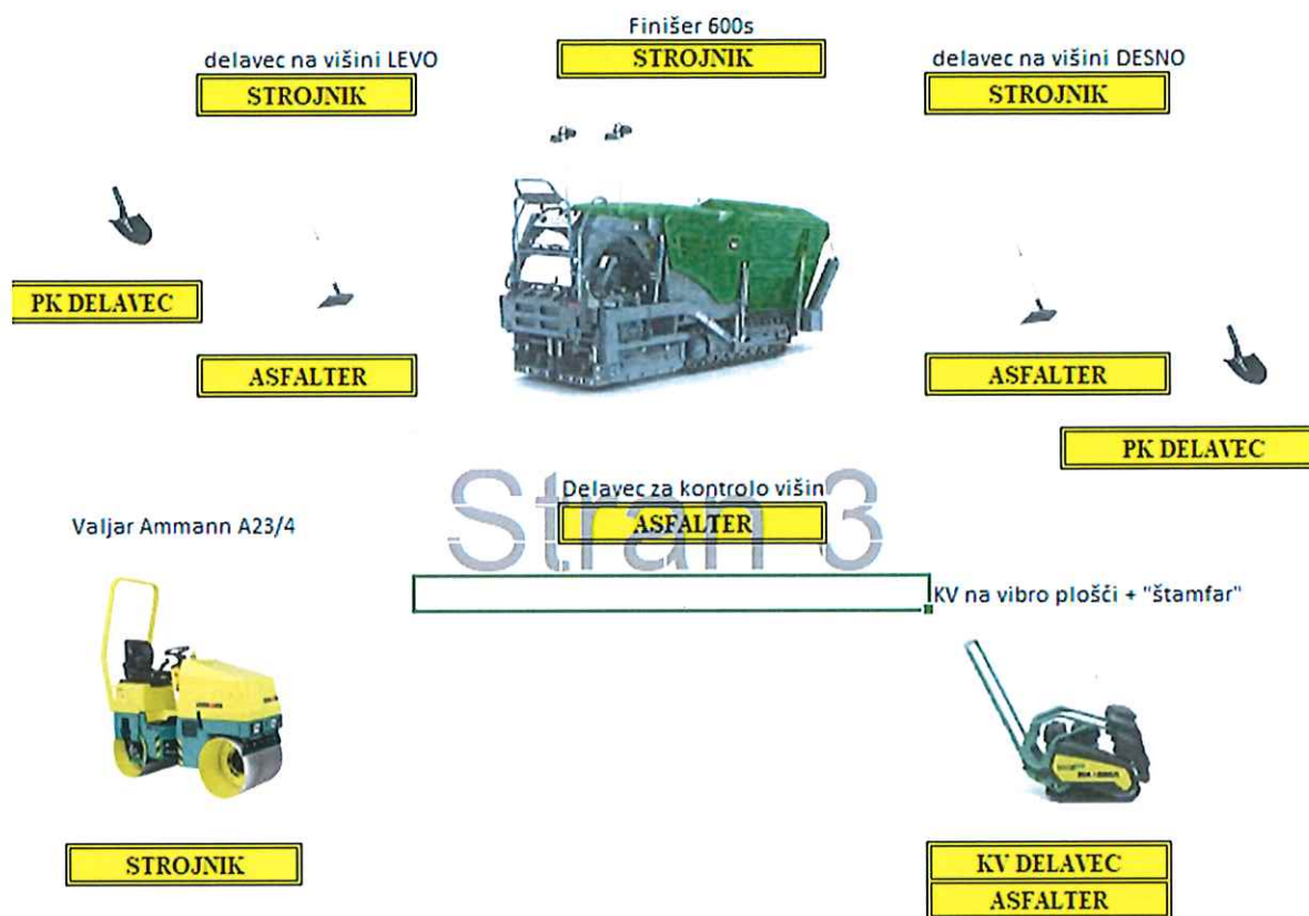
Slika 5: vgradnja asfalta z malim finišerjem od 20 – 100 m 2
