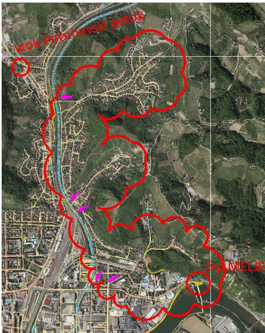
Slika 4: Območje obdelave, kjer je potrebno urediti kanalizacijo za odpadne vode
