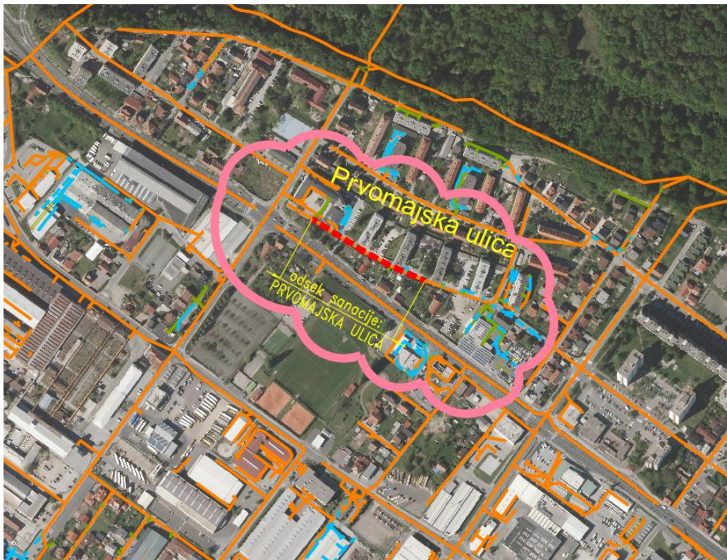
Slika 1: Pregledna situacija odseka Radvanjske ceste, kjer je predvidena sanacija kanalizacijskega omrežja
