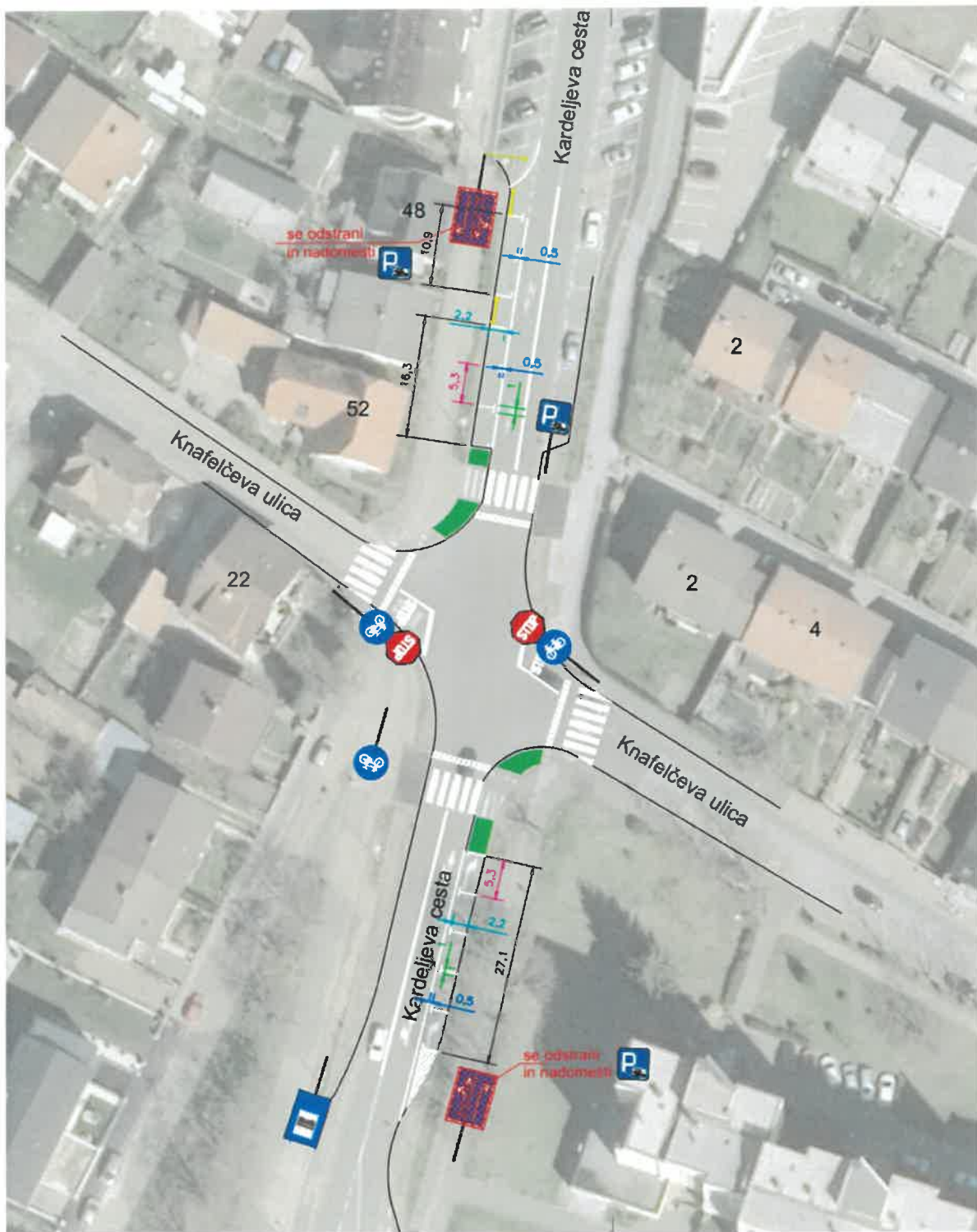
Slika 1: Gradbena situacija
