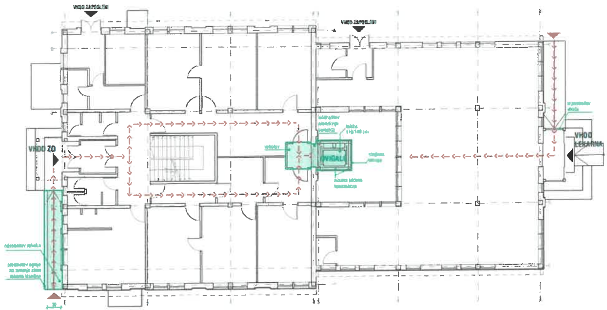
Slika 6: Tloris pritličja s predlagano umestitvijo dvigala
