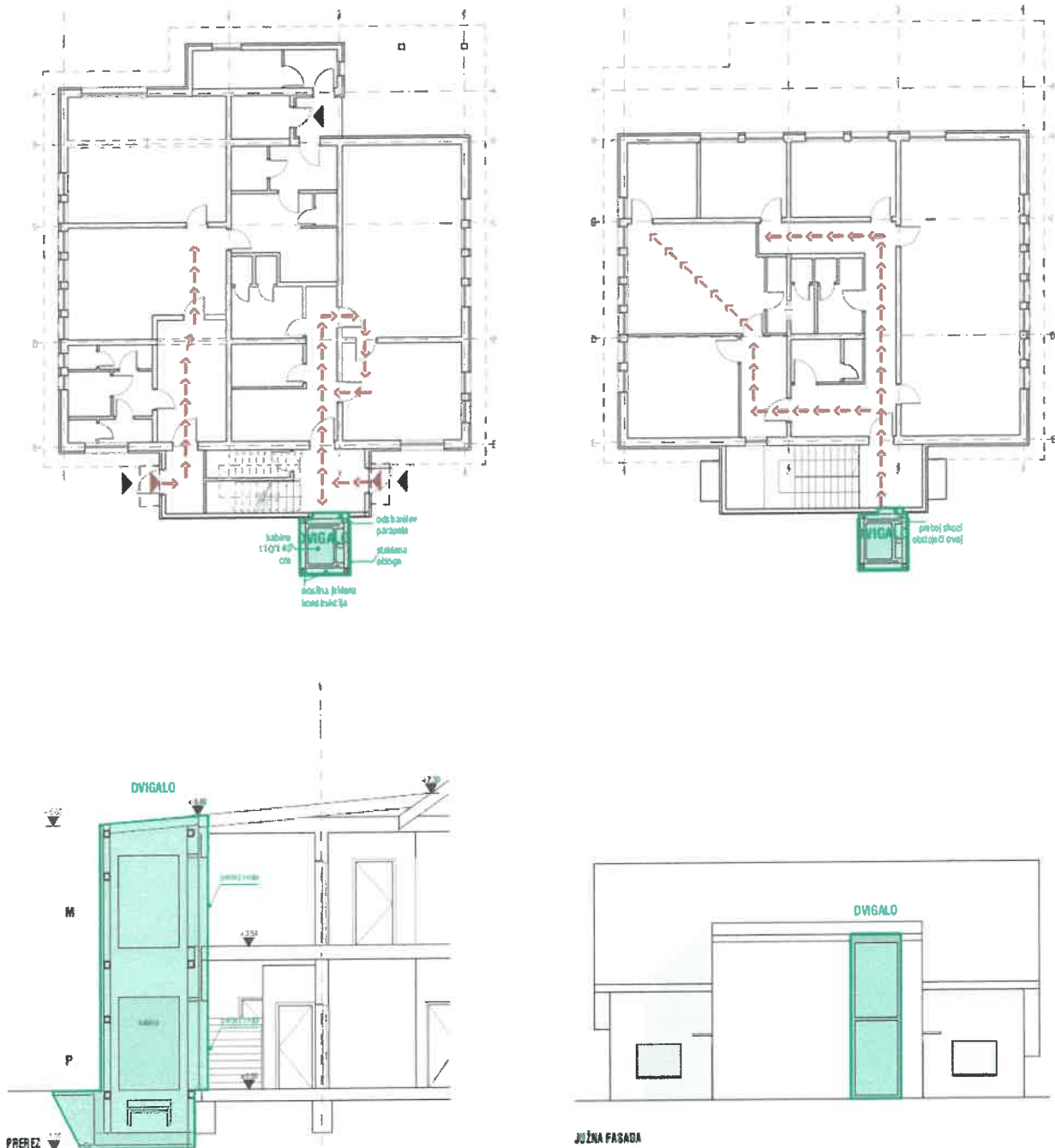
grafika: PREREZ IN FASADA _m 1:75, 1:125
