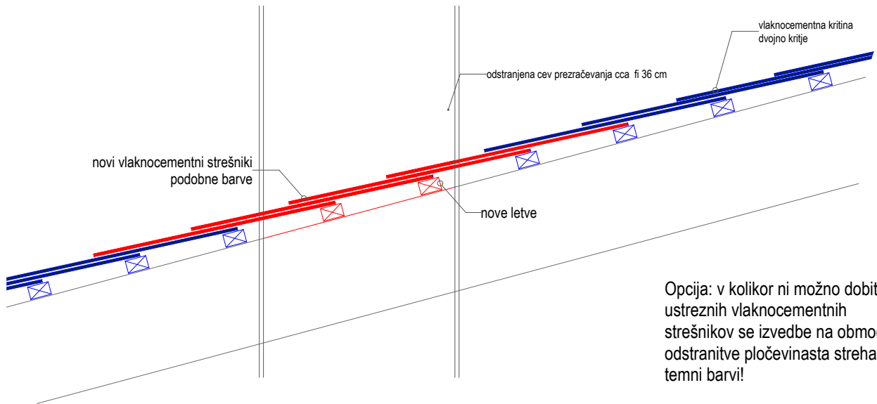
ZASNOVA KR PANJA STREHE PO ODSTRANITVI PREZRAČEVANJA / PREREZ
